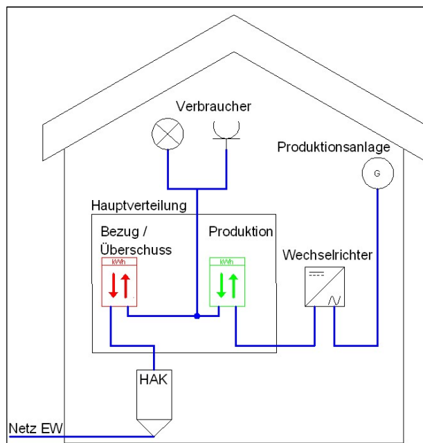
Abbildung 1: Schema Eigenverbrauchsmodell
